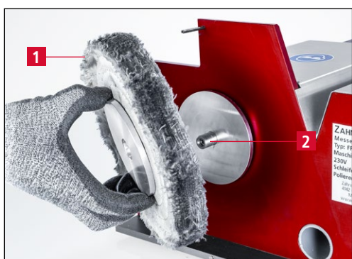
Figure 7-14 Retirer la bride de serrage et le disque de polissage
