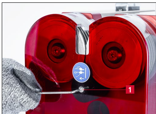
Figure 7-6 Dévisser la vis de fixation du capot de protection des meules en spirale
