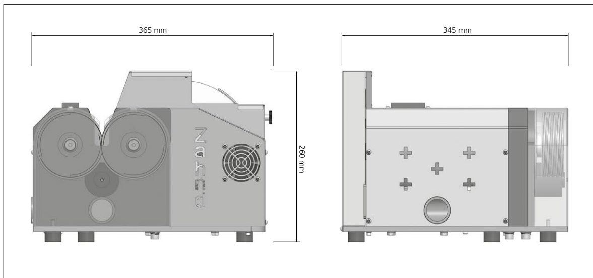
Figure 3-1 Dimensions en mm
